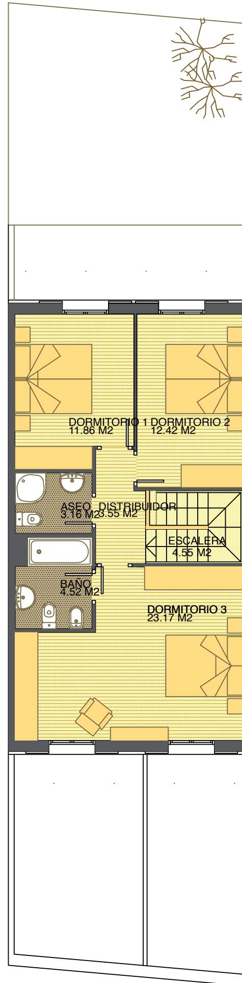
PLANTA PRIMERA SUPERFICIE UTIL VIVIENDA: 63.128 M 2 .
