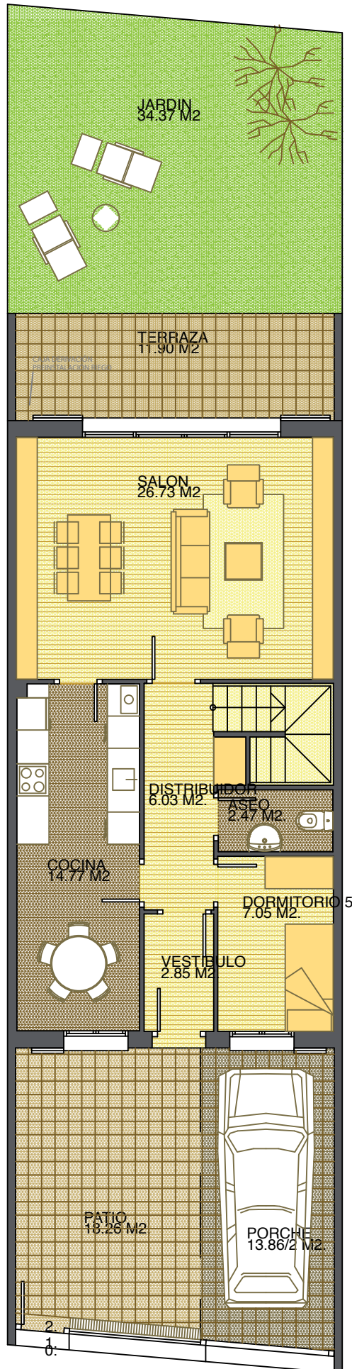
PLANTA BAJA SUPERFICIE UTIL VIVIENDA 59.90 M 2 . SUPERFICIE UTIL PORCHE 13.86/2 M 2 .
