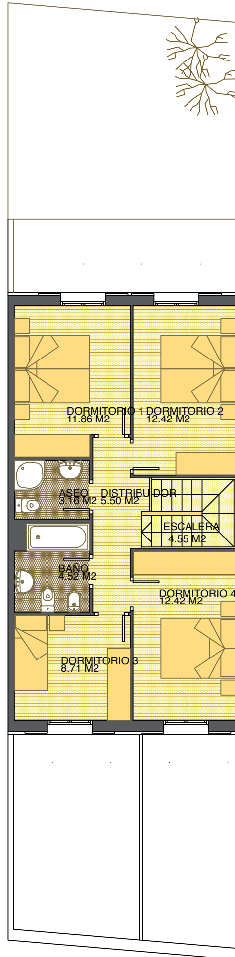
PLANTA PRIMERA SUPERFICIE UTIL VIVIENDA 63.14 M 2 .
